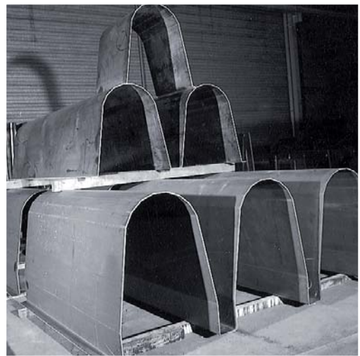
geplooidetrogvormen lengte 4000 mm dikte 8 mm geplooide hoogte 1400 mm
